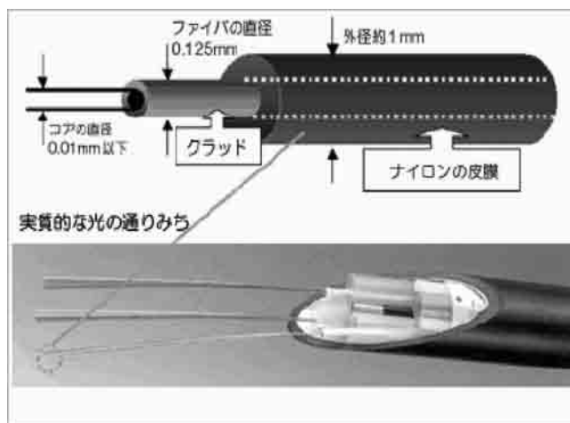
光ファイバー構造図
